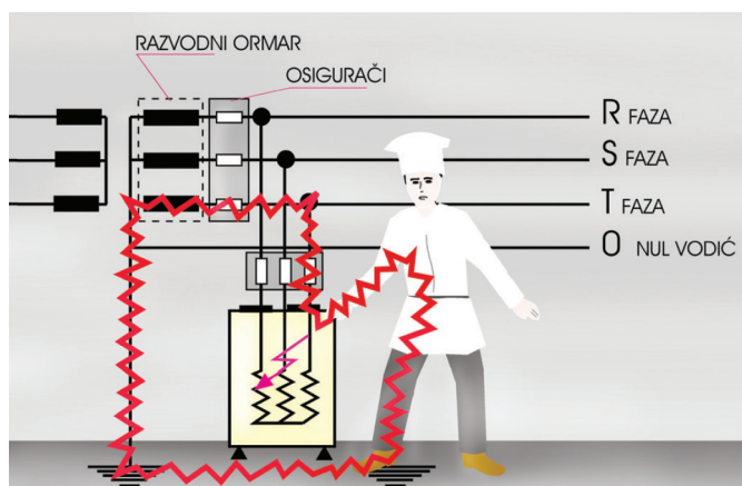
Sl. 5. Indirektni napon dodira nastaje kada metalno kućište koje inače nije pod naponom- npr. bojler, električni štednjak i sl. uslijed proboja izolacije i sl. dođe pod napon (napon greške). Što je manji otpor prolasku električne struje kroz tijelo čovjeka i veći napon na kućištu, kroz čovjeka prolazi jača struja prema poznatom izrazu I = U/R . ( I jakost struje u amperima, U je napon u voltima te R otpor u omima). Važno je i vrijeme trajanje udara. Smrt može nastupiti kada je napon izmjenične struje veći od 50 V (u normalnim uvjetima), ali i kod manjeg napona u ekstremnoj vlažnosti i dodira s metalom po većoj površini tijela.
