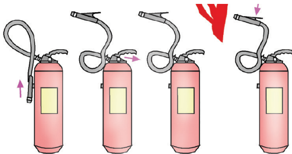
Sl.32. Postupak aktiviranja aparata za početno gašenje požara: 1. donjeti aparat na prihvatljivu udaljenost od požara, uhvatiti mlaznicu, 2. izvući osigurač, 3. usmjeriti mlaznicu prema požaru, 4. pritisnuti ručicu na aparatu i ručicu na mlaznici na crijevu (ukoliko je izvedena)
