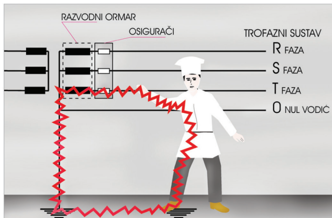
Sl. 4. Strujni udar uslijed direktnog napona dodira čovjek je dotaknuo tzv. fazu sustava koja ima napon prema zemlji 220 V pri čemu se preko tijela zatvara strujni krug.
